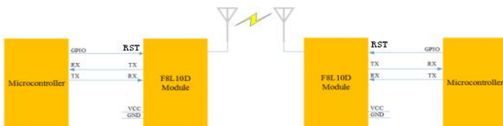
图 3-2 两个模块互相通信指示图
